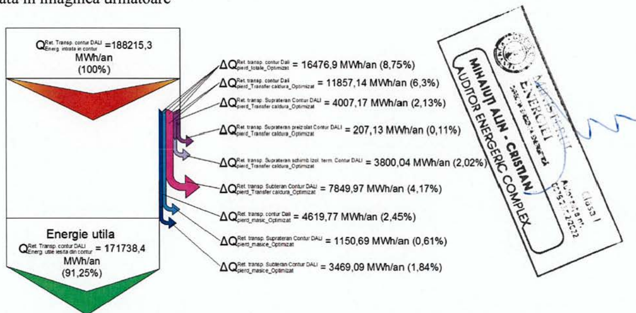
Diagrama Sankey – Bilant termoenergetic anual optimizat pentru sistemul de transport cuprins in documentatia DALI – (conturul analizat)
